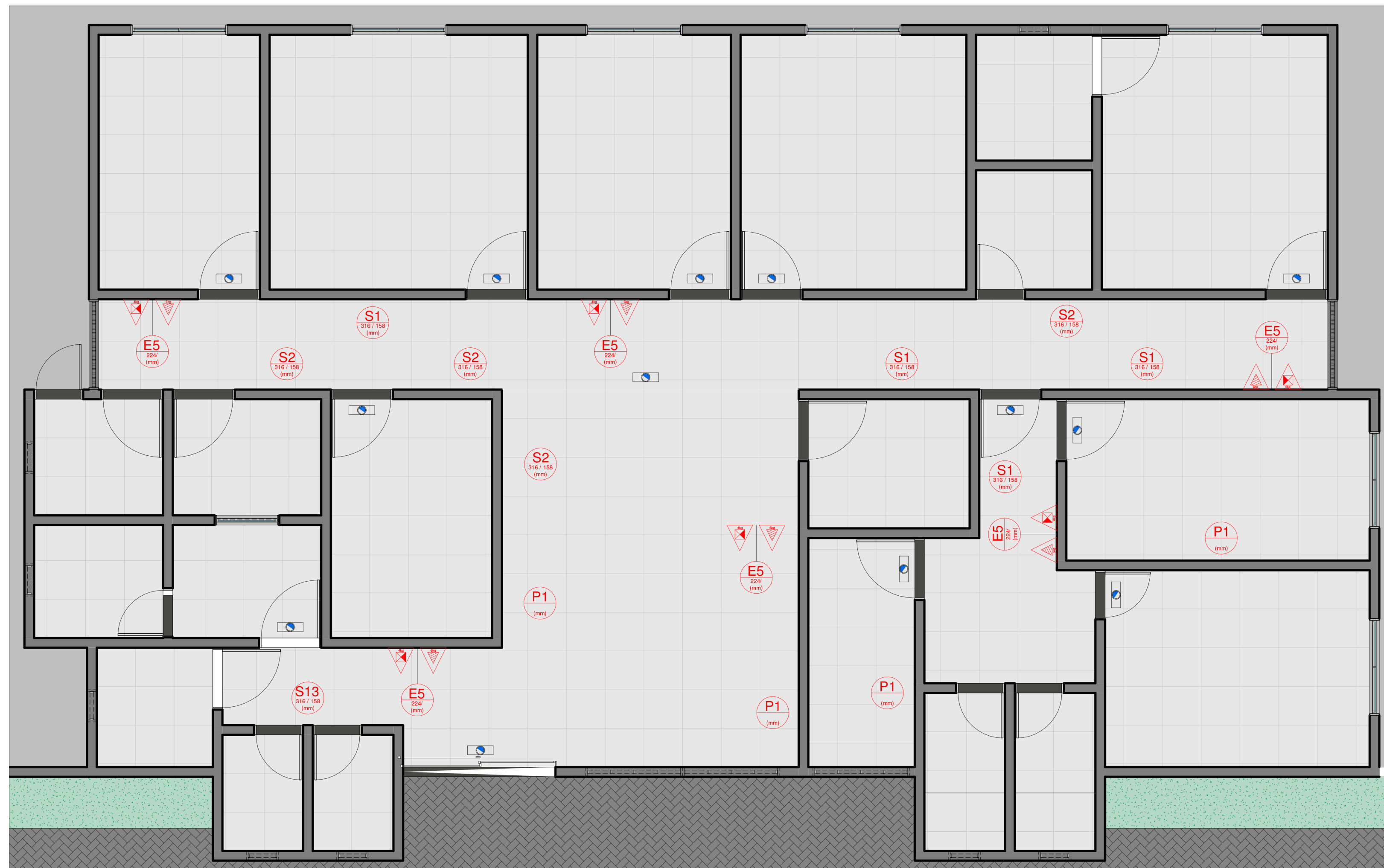
1 PLANTA DE EMERGÊNCIA ESCALA 1:50
